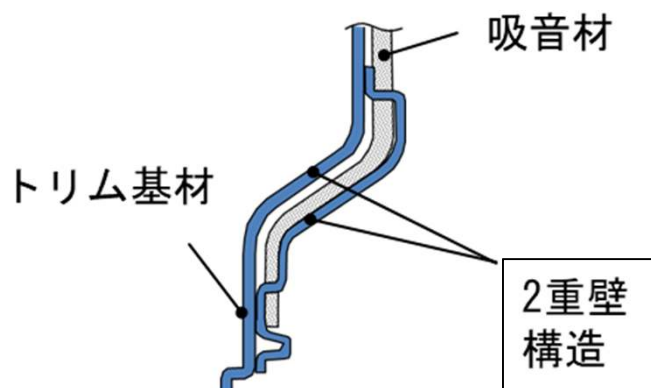
新製品(2重壁構造)の断面図
